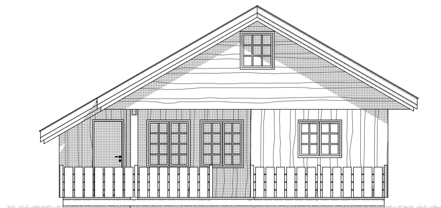
Fasade sydøst
